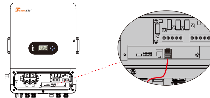
Рис. 4.6-2 Інтерфейс RJ45
